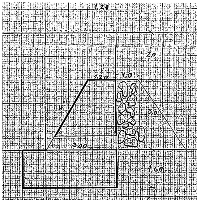
Слика 1: Попречни пресек
