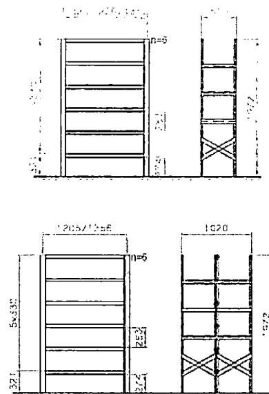
Karakterističan pogled na polja jednoređnih i dvoređnih regala
